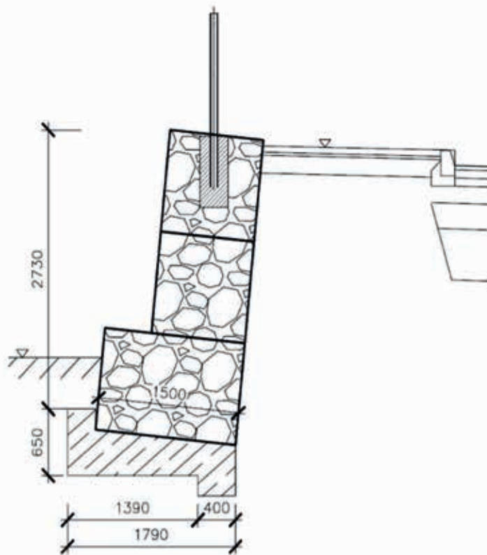
Obr. 5. Schematický tvar gabionové tížní zdi
